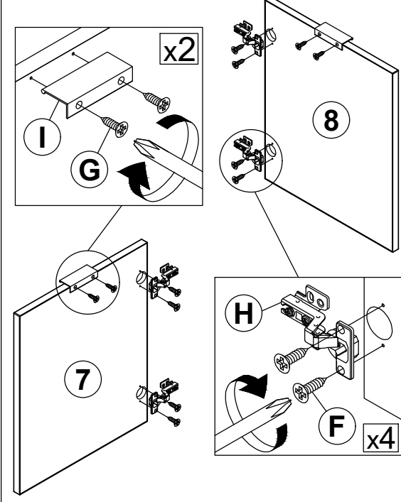
Step 15
